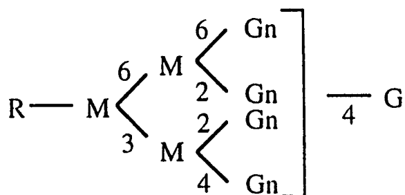
M 3 Gn 4 G. Tetra-antennary complex
